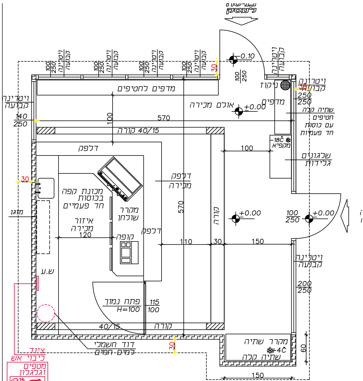
סידור פנים ק.מ.:1:50 קומת קרקע
